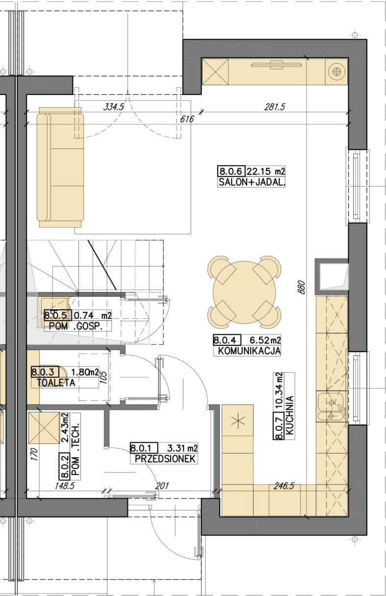
RZUT PARTERU
