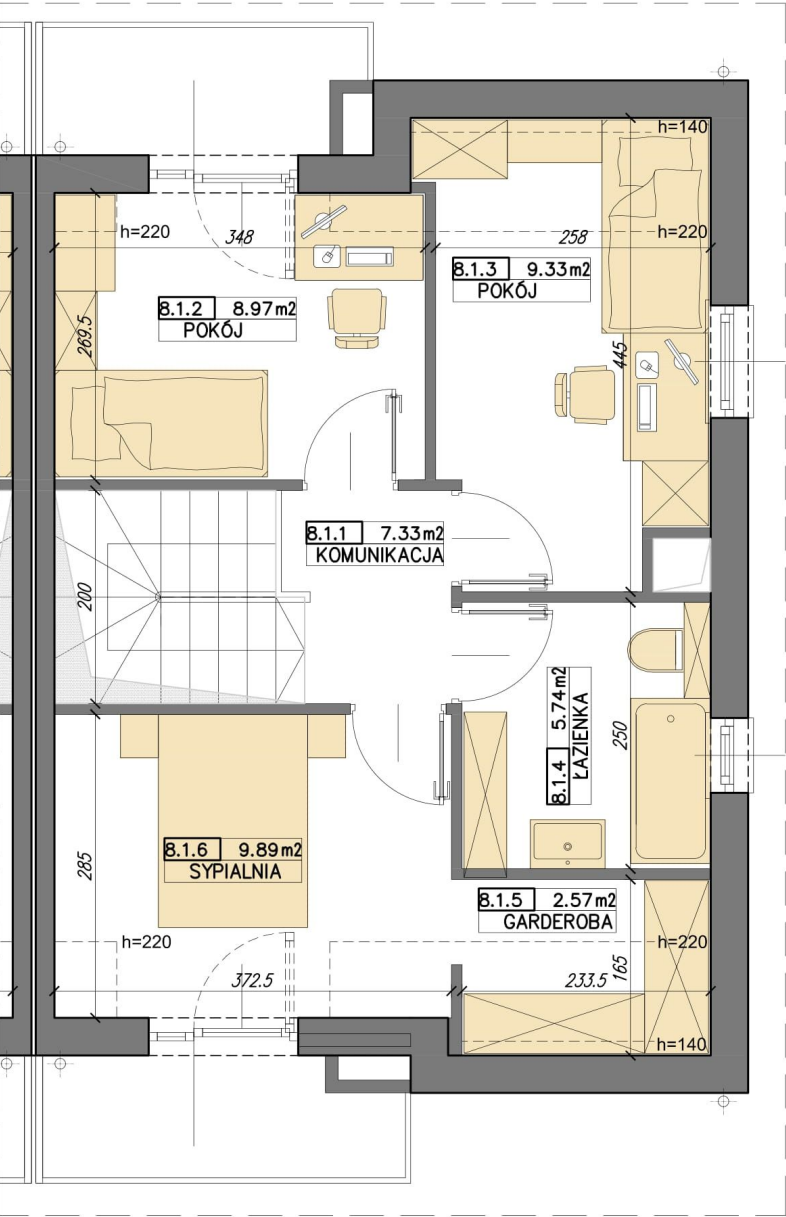
RZUT PIĘTRA
